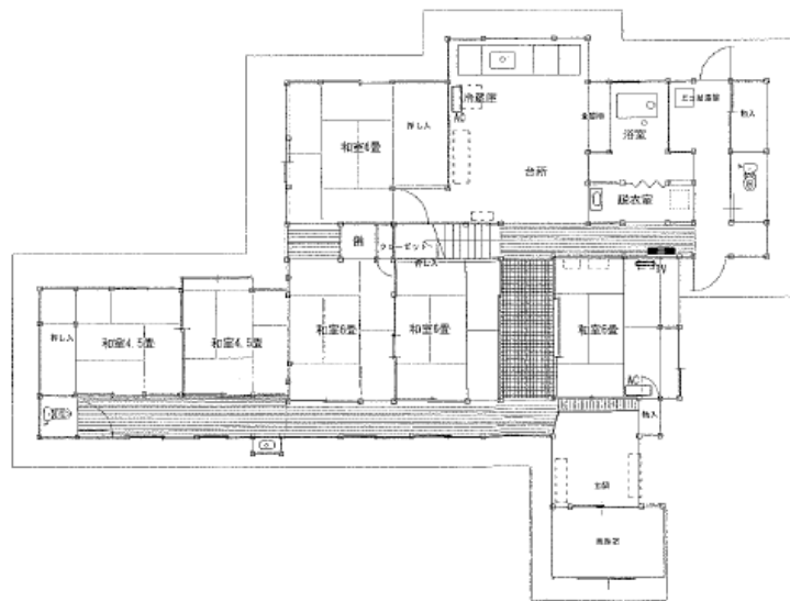
1階平面図
